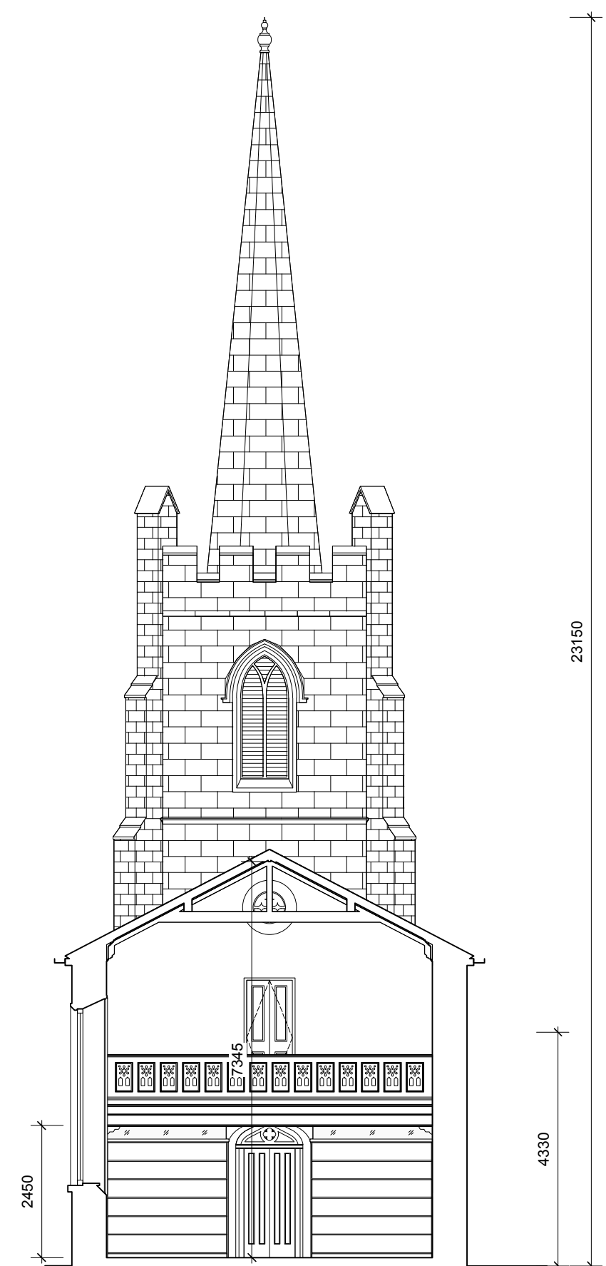
SECTION A-A
