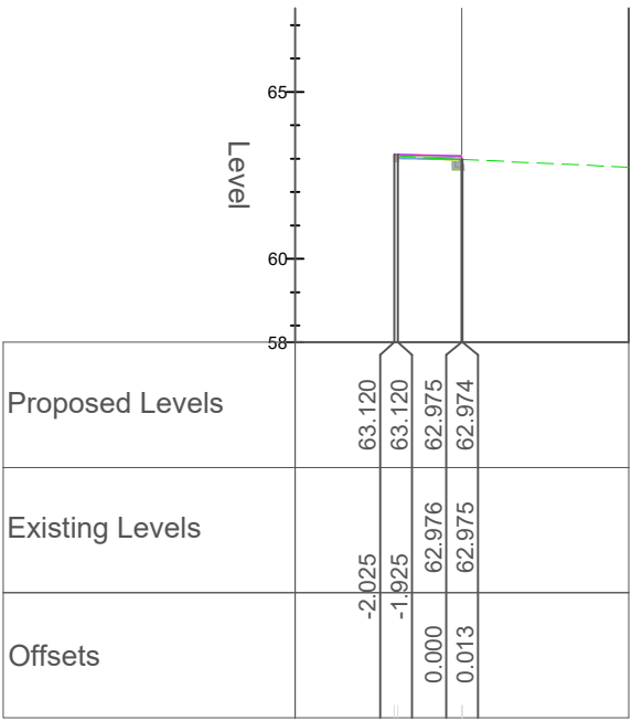
Chainage 60.000 (124)
