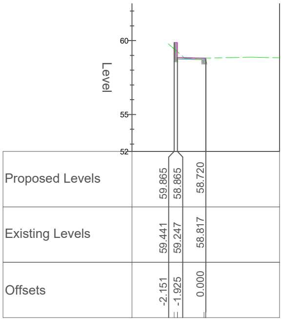
Chainage 240.000
