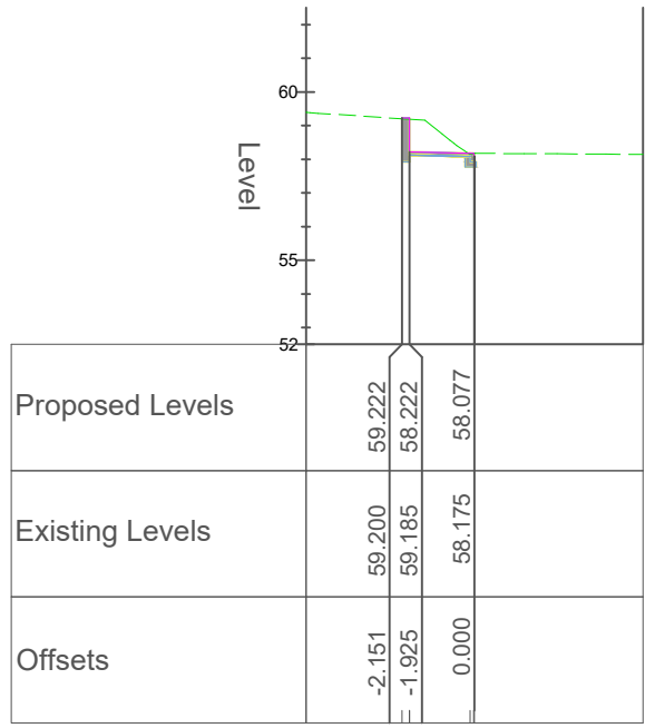
Chainage 200.000
