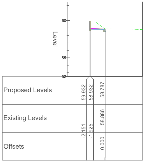
Chainage 220.000
