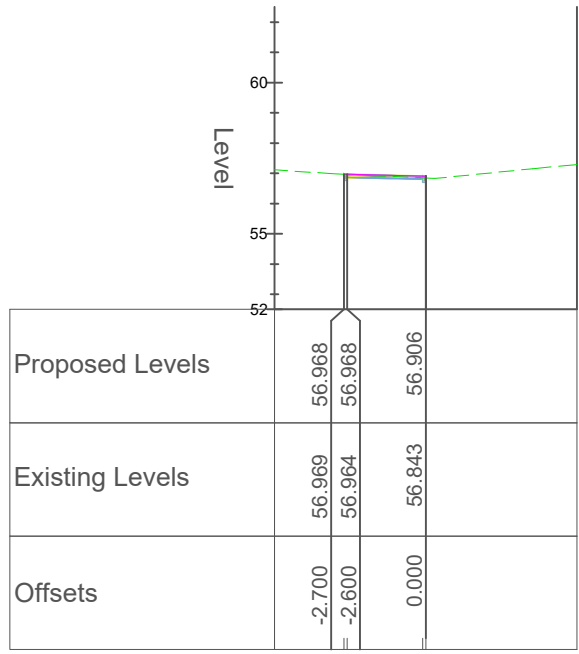
Chainage 160.000
