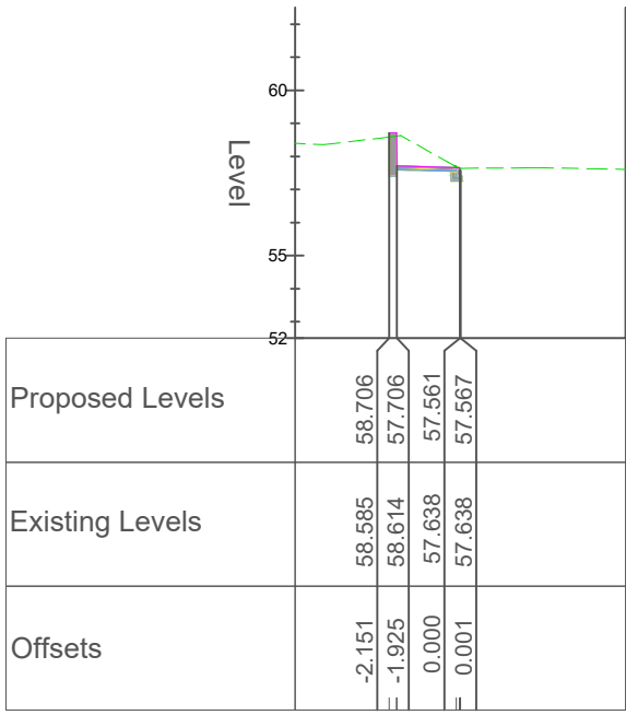
Chainage 190.000
