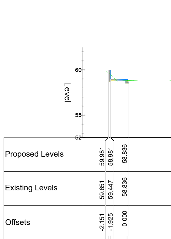
Chainage 240.000
