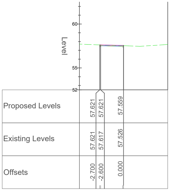
Chainage 170.000
