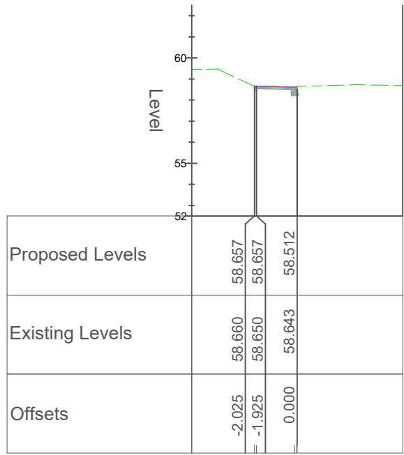
Chainage 260.000
