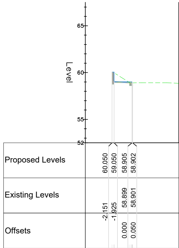
Chainage 230.000
