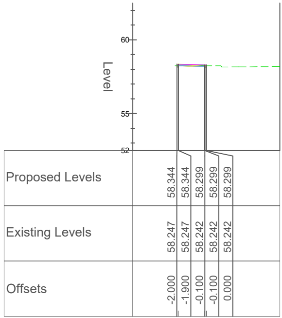
Chainage 330.000
