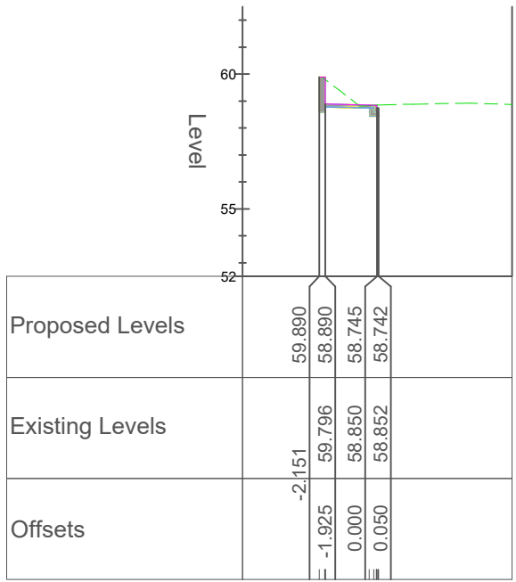
Chainage 230.000
