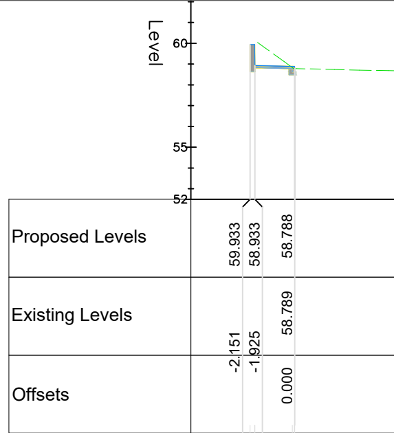
Chainage 220.000
