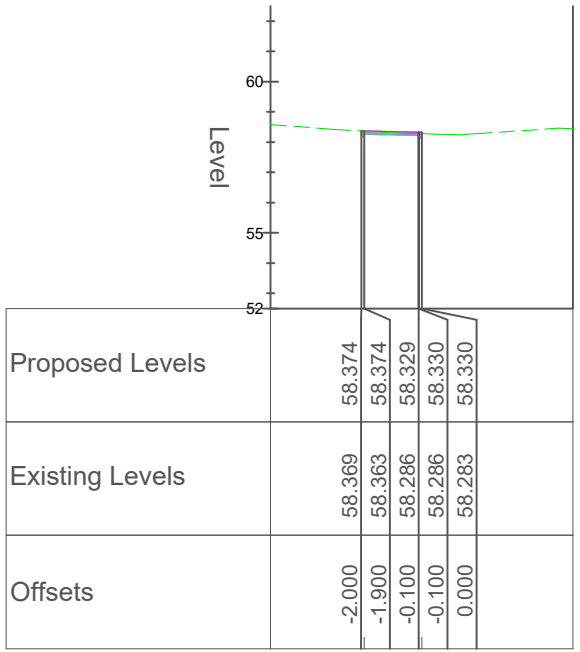
Chainage 300.000
