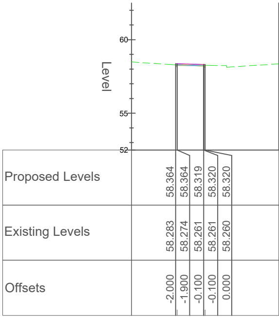
Chainage 310.000
