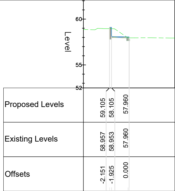
Chainage 200.000
