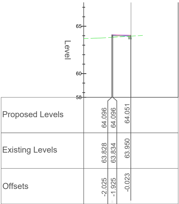
Chainage 0.000
