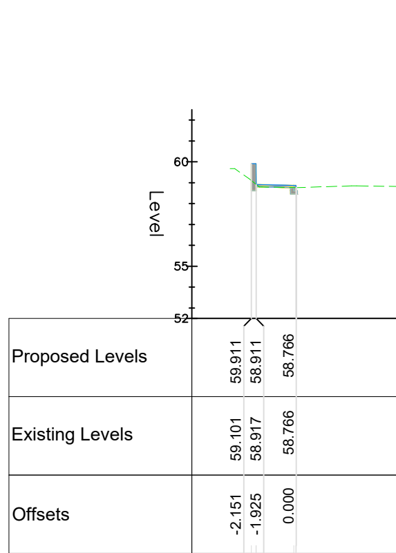
Chainage 250.000
