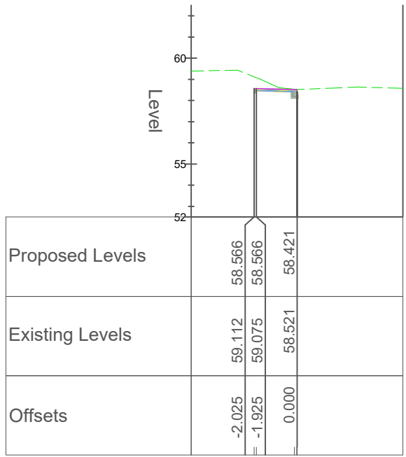
Chainage 270.000
