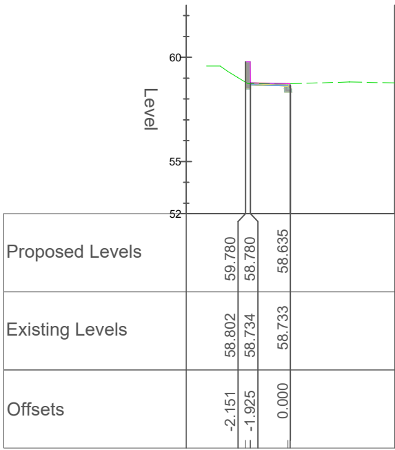
Chainage 250.000
